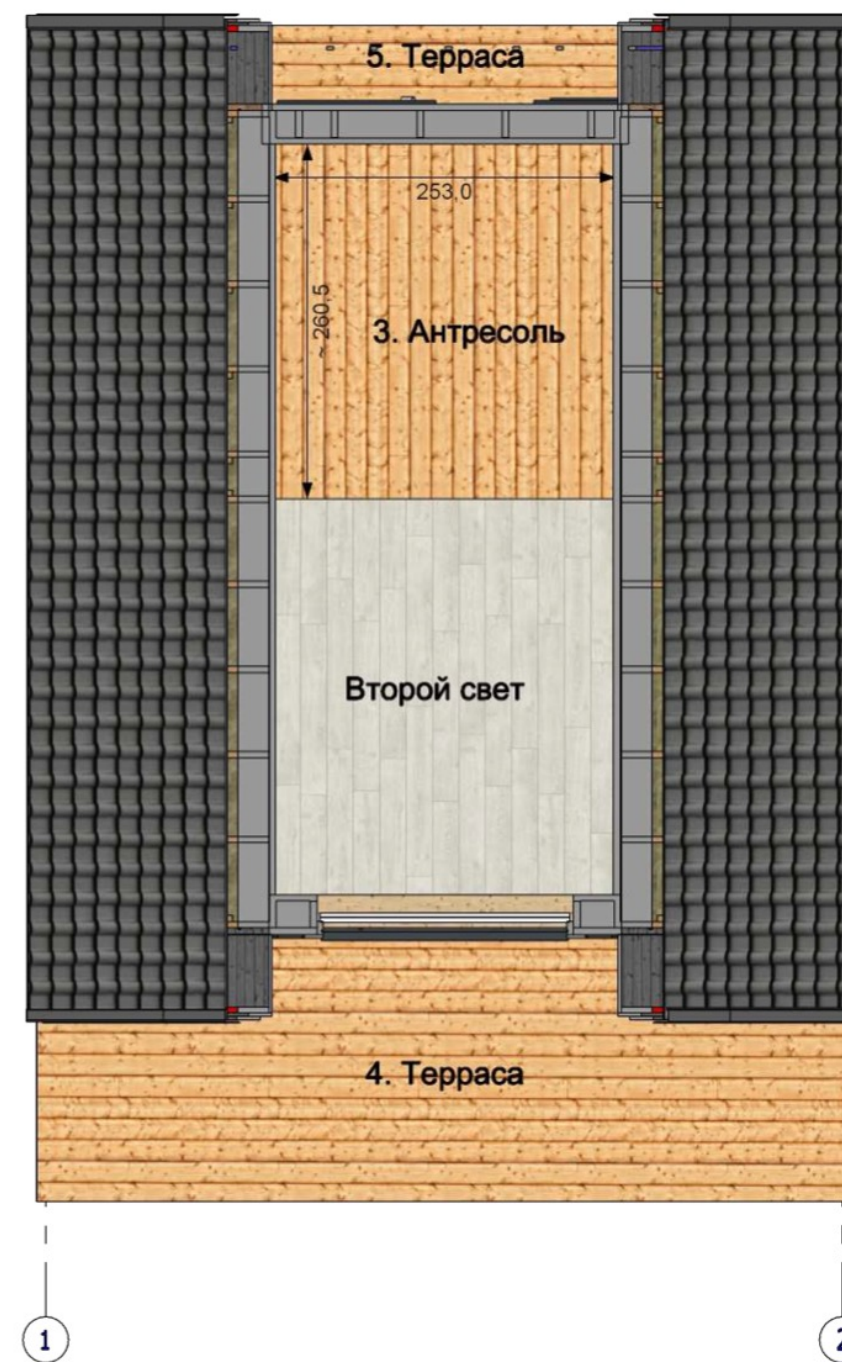
Планировка 2 этаж
